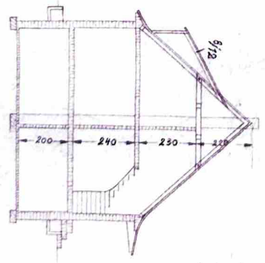
Schnitt 7/4 Schiefer 1/4 Zangen 2x1/8
